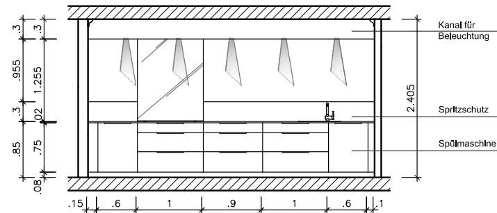
Wandansicht A1, M 1:50
