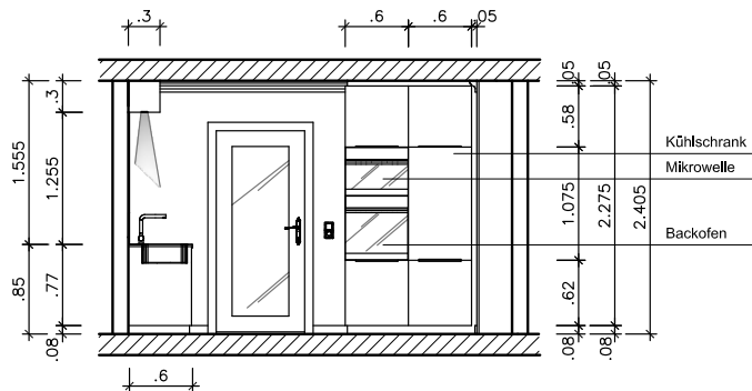
Wandansicht B, M 1:50
