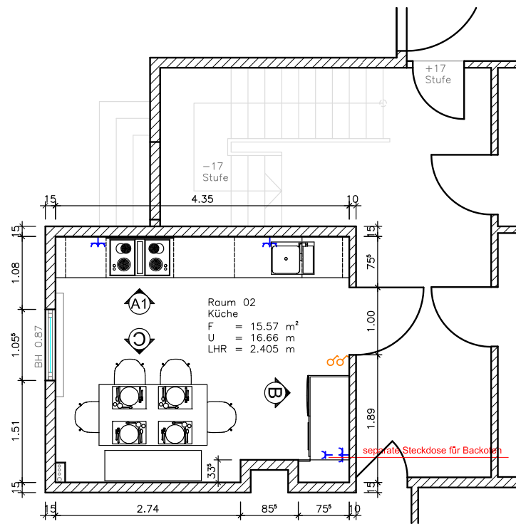
Grundriss Variante 1 > Dunstabzug versenkbar, M 1:50
